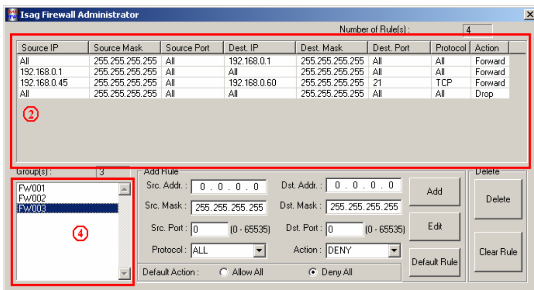
รูปที่ 15 แสดงการเลือกกลุ่มที่ต้องการลบกฎการฟิเตอร์ทั้งหมดและรายการกฎของกลุ่มทั้งหมด
