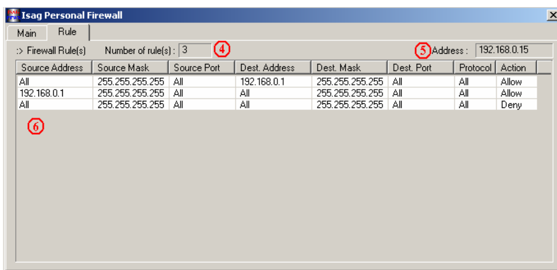
รูปที่ 27 แสดงส่วนต่างๆ ของหน้า Rule ของโปรแกรม ISAG Personal Firewall
