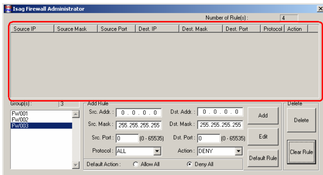
รูปที่ 17 แสดงกฎการฟิเตอร์ของกลุ่มที่ถูกลบทั้งหมดแล้ว
