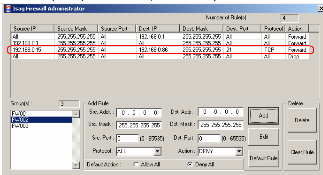
รูปที่ 6 แสดงกฎการฟิเตอร์ที่ถูกเพิ่มเข้าไปให้กลุ่ม
