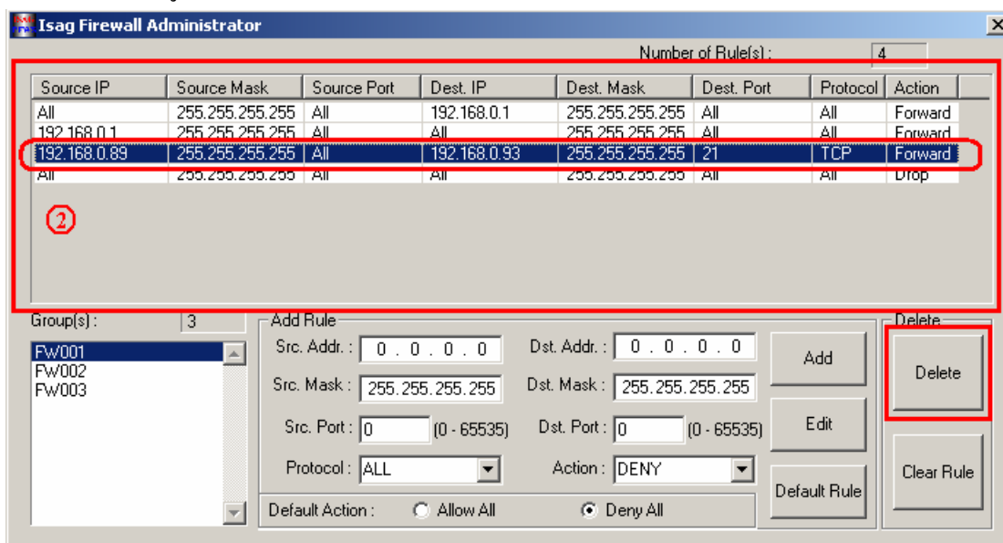
รูปที่ 13 แสดงการเลือกกฎที่ต้องการลบและปุ่มลบกฎ
