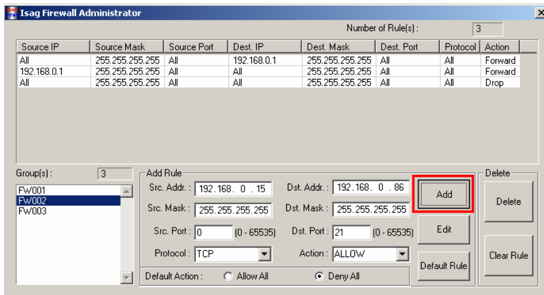
รูปที่ 5 แสดงการกดที่ปุ่ม Add เพิ่มเพิ่มกฎที่กำหนดไว้เข้ากลุ่ม
