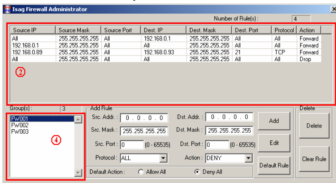
รูปที่ 12 แสดงการเลือกกลุ่มและรายการกฎของกลุ่มที่เลือก
