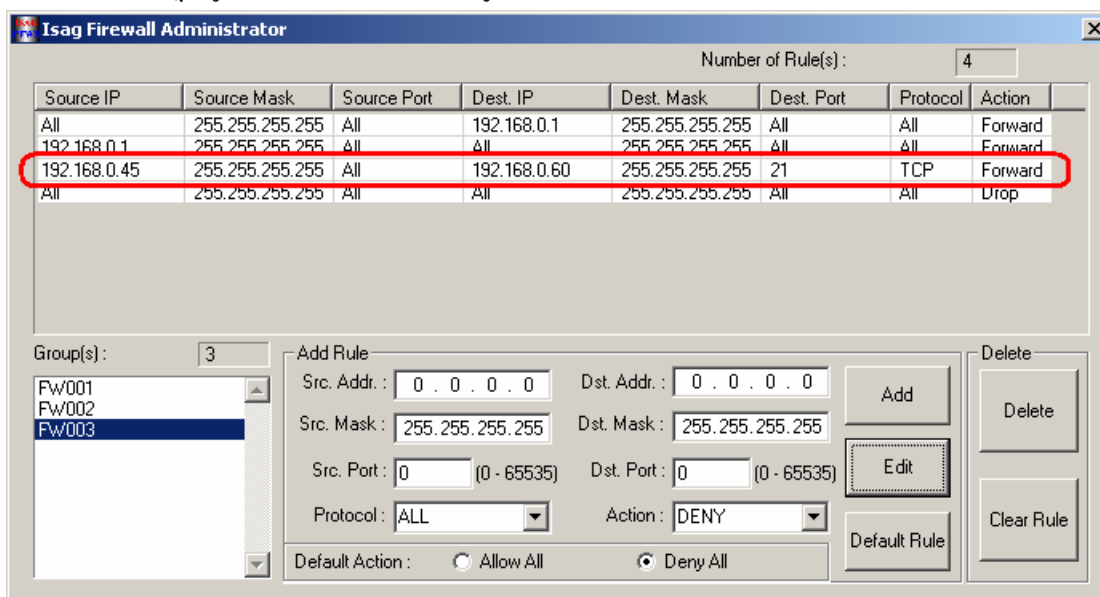
รูปที่ 11 แสดงกฎที่ถูกแก้ไขเรียบร้อยแล้ว
