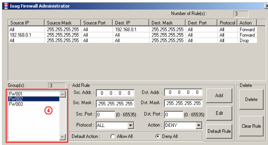
รูปที่ 3 แสดงการเลือกกลุ่มที่ 2 ที่ส่วนที่ 4
