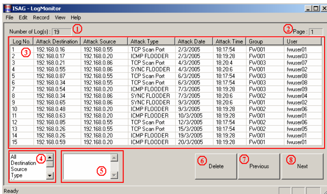
รูปที่ 19 แสดงส่วนต่างๆ ของโปรแกรม ISAG Log Monitor
