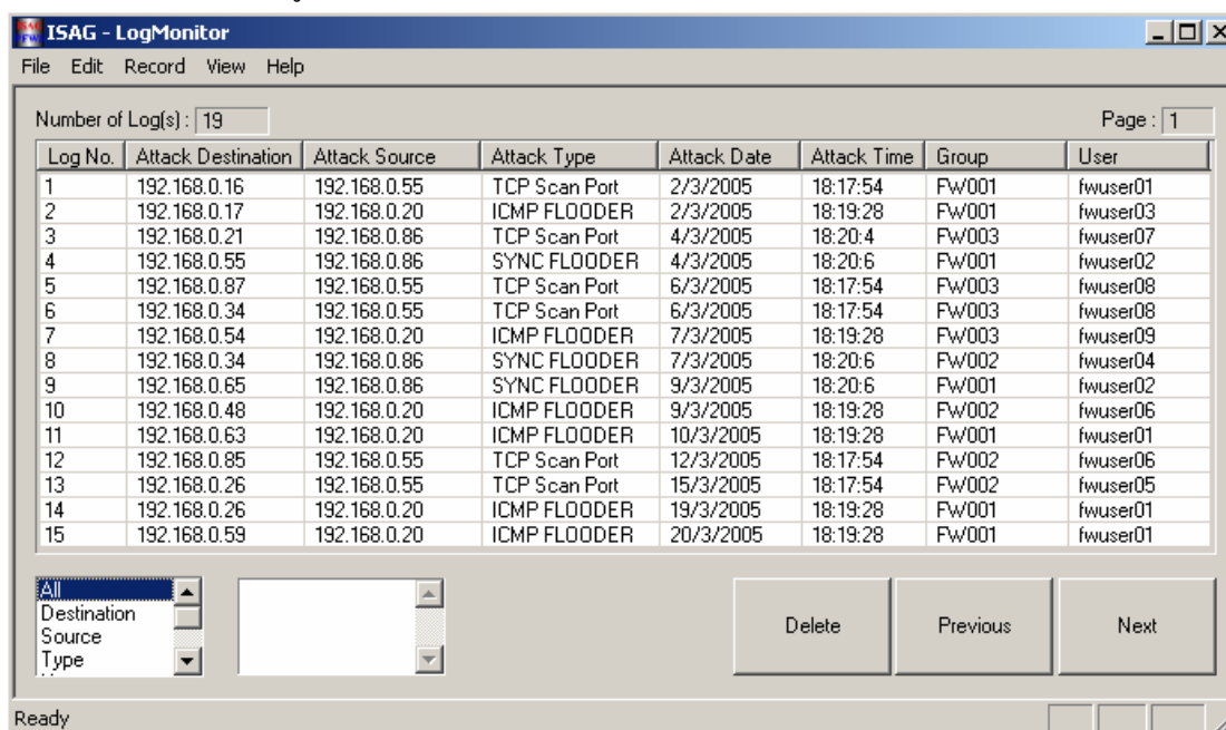
รูปที่ 22 แสดงรายการข้อมูลทั้งหมด
