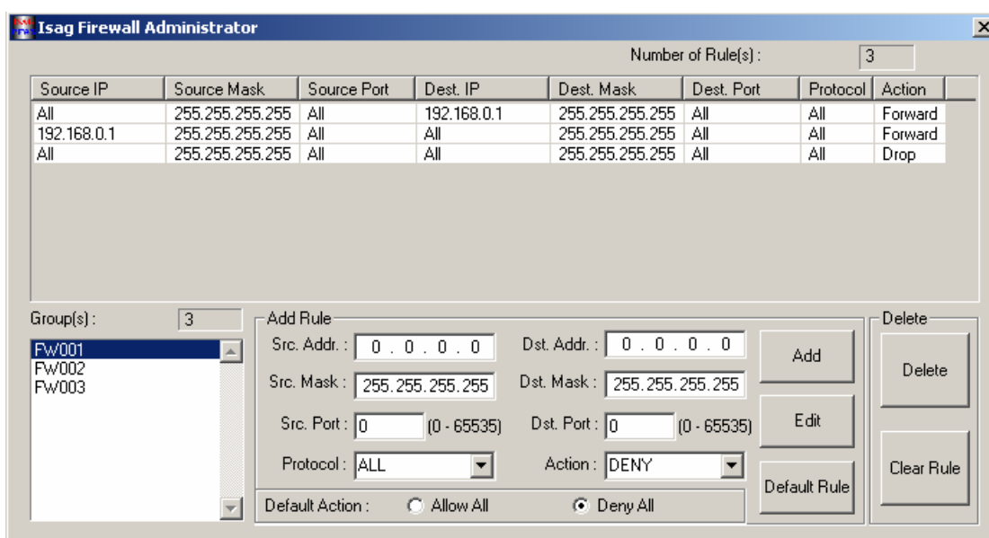
รูปที่ 1 แสดงรูปเมื่อเริ่มเปิดโปรแกรม Isag Firewall Administrator ขึ้นมา
