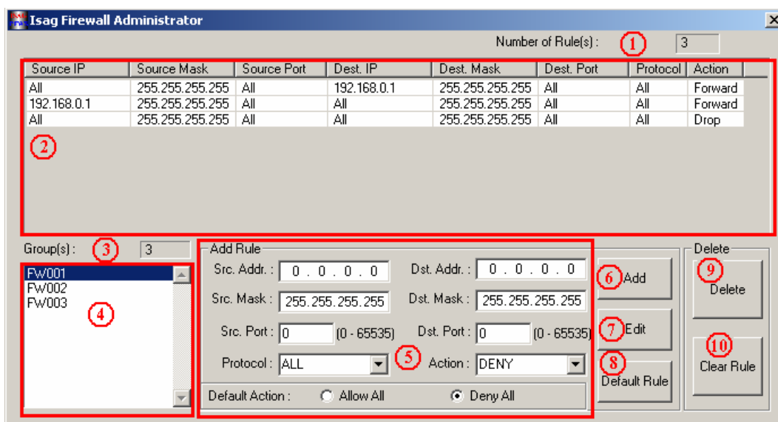
รูปที่ 2 สำหรับอธิบายส่วนต่างๆของโปรแกรม
