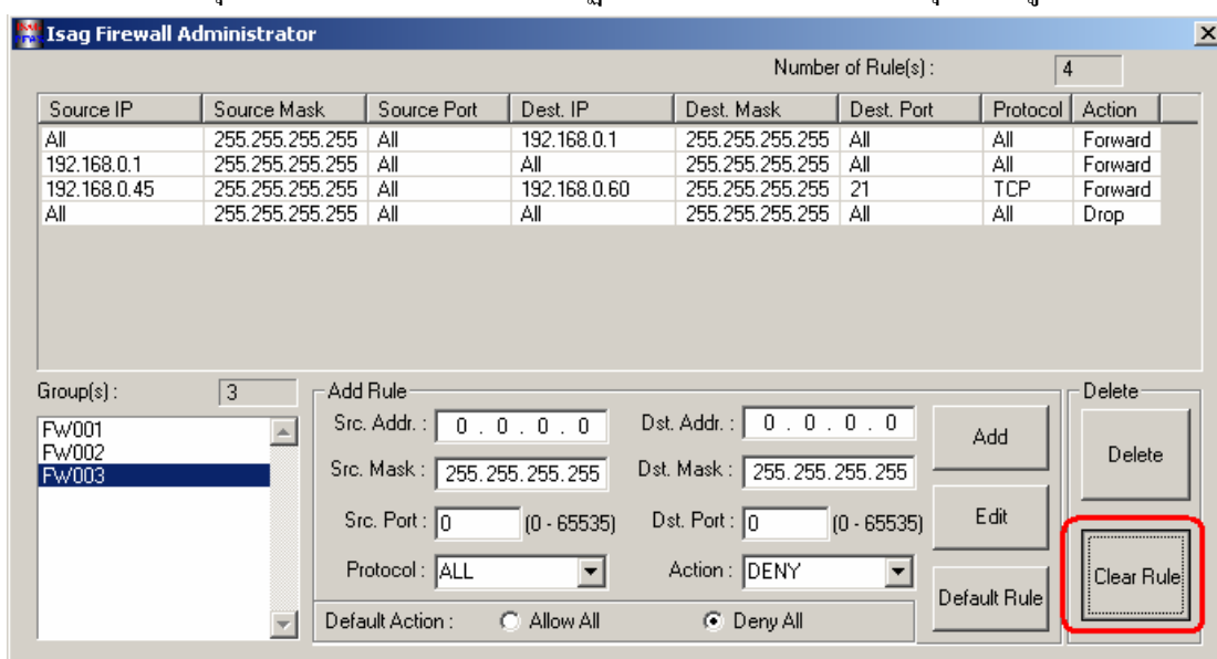
รูปที่ 16 แสดงการกดปุ่ม Clear Rule เพื่อลบกฎการฟิเตอร์ทั้งหมดของกลุ่ม
