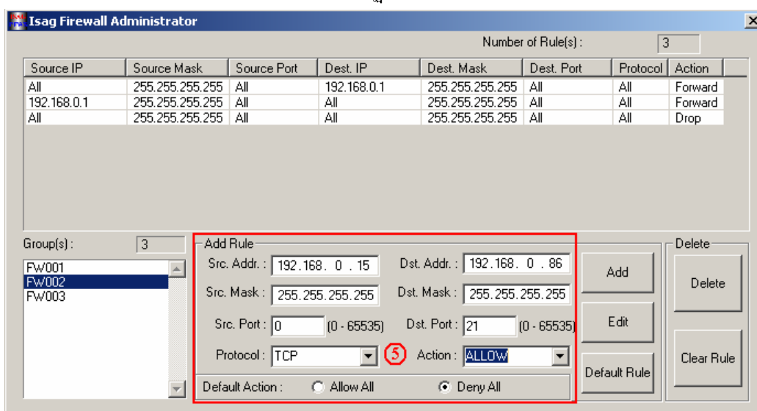
รูปที่ 4 แสดงการตั้งค่าต่างๆ ในส่วนที่ 5 เพื่อเพิ่มเป็นกฎการฟิเตอร์
