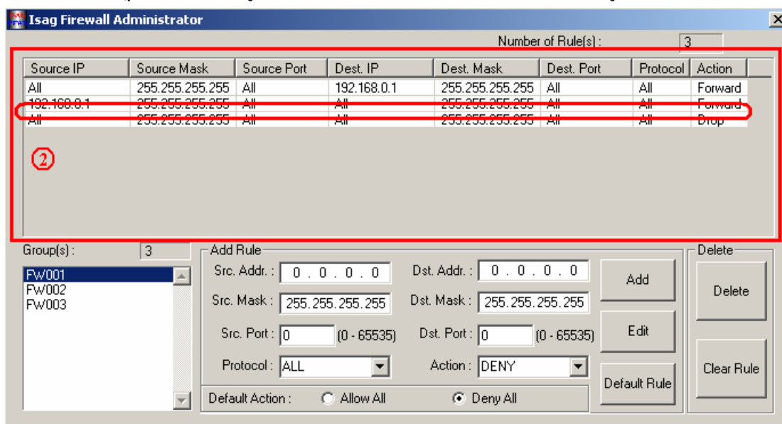
รูปที่ 14 แสดงกฎการฟิเตอร์ที่เหลือหลังจากลบไปแล้ว
